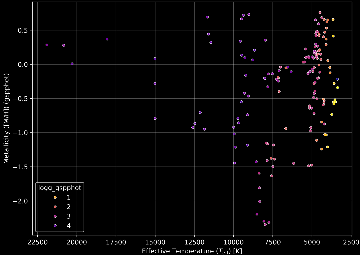
APOGEE DR17 Field: [075+00] Stellar Population Parameters (n= 159)
